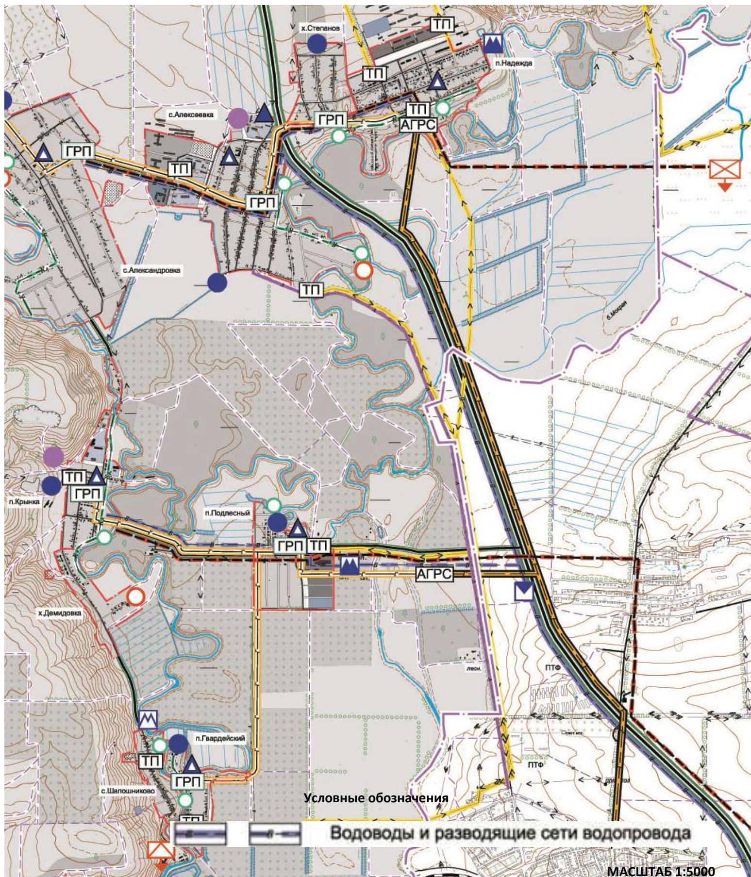
Схема существующего и планируемого водопровода Алексеевского сельского поселения
